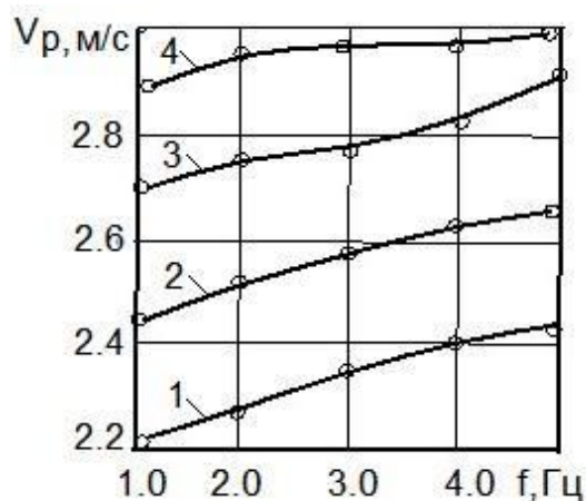
Рисунок 6 – Залежність швидкості активного рихлення породного масиву S=100 на глибину 0,4 м від частоти ударів: 1, 2, 3, 4 – при енергії ударів відповідно 6,0; 7,0; 8,0; 9,0 кДж і тягловому зусиллі 0,16 МН
