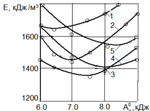
Рисунок 10 – Залежність питомої енергоємності активного рихлення від енергії удару: 1, 2, 3, 4 і 5 – при рихленні на глибину відповідно 0,4; 0,5; 0,6; 0,7 і 0,8 м
