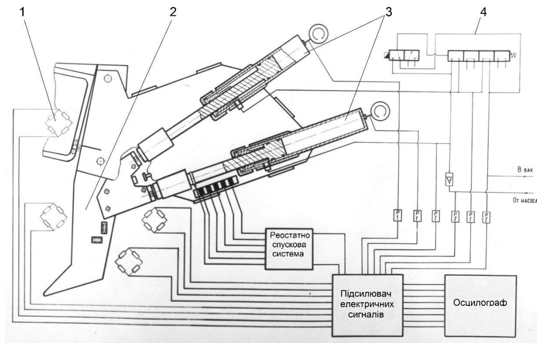
Рисунок 3 – Повнорозмірний випробувальний стенд активного розрихлювача: 1 – тензометричні датчики; 2 – зуб розрихлювача; 3 – гідропневмоударники; 4 – гідросистема управління
