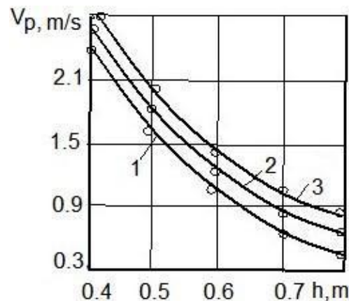
Рисунок 4 – Залежність швидкості активного розрихлювача від глибини рихлення мерзлого ґрунту VIII: 1, 2, 3 – при енергії одиничного удару відповідно 6,0; 7,0; 8,0 кДж
