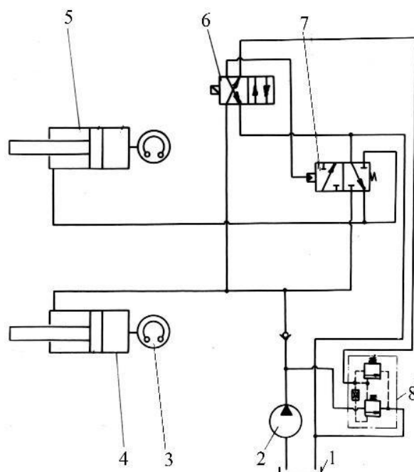
Рисунок 2 - Гідравлічна схема динамічного вузла активного розрихлювача: 1 – бак з робочою рідиною; 2 – гідронасос; 3 – пневмоакумулятор; 4 – нижній гідропневмоударник; 5 – верхній гідропневмоударник; 6, 7 – гідророзподільники; 8 – золотник управління
