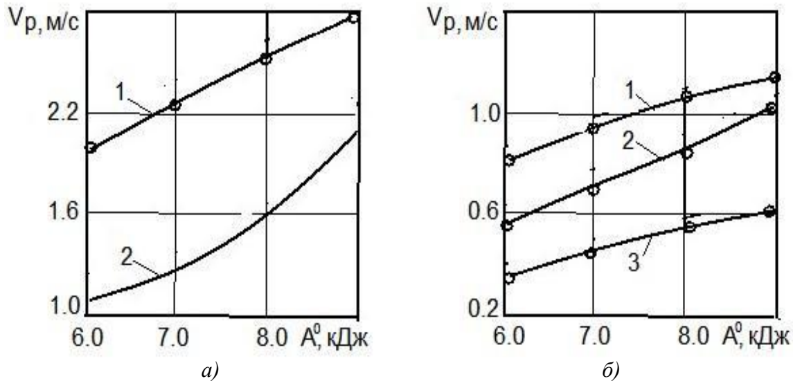
Рисунок 7 – Залежність швидкості активного розрихлювача від енергії удару: а - при рихленні на глибину 0,4 м (1) і 0,5 м (2); б – при рихленні на глибину 0,6 м (1), 0,7 м (2) і 0,8 м (3)
