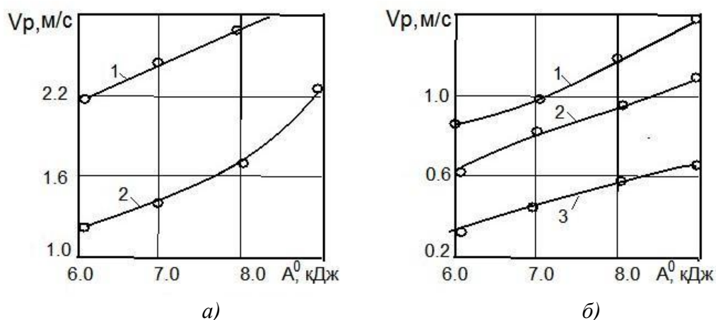
Рисунок 5 - Залежності швидкості активного розрихлювача від енергії удару:
