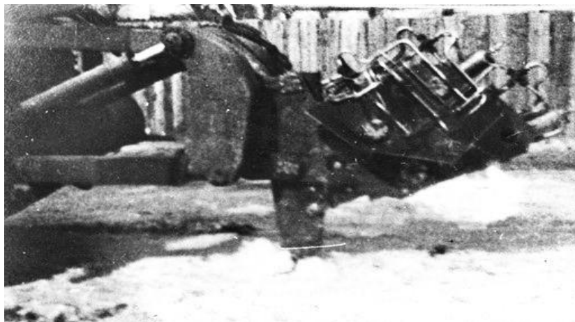
Рисунок 12 – Динамічна приставка до статичного розрихлювача
