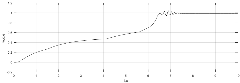
Рисунок 4 – Графік переходного процесу за швидкістю при пуску
