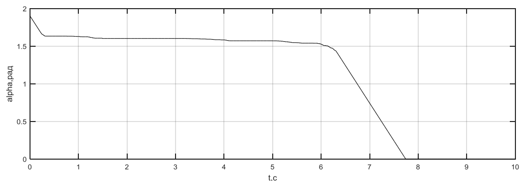
Рисунок 6 – Графік переходного процесу за кутом відпирання при пуску
