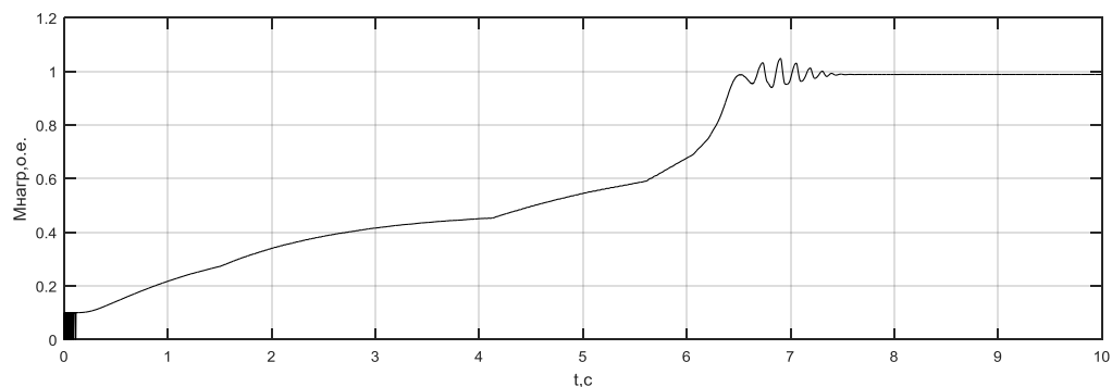
Рисунок 5 – Графік переходного процесу за моментом навантаження при пуску
