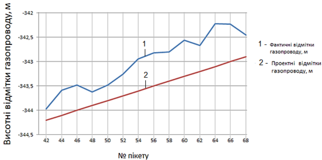
Рисунок 3 – Характерні ділянки зміни профілю траси трубопроводу в зонах інтенсивного здимання порід підосви виїмкового хідника шахти «Тернівська»
